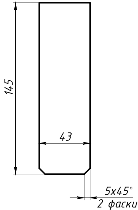
Поз.2 (Ребро)
