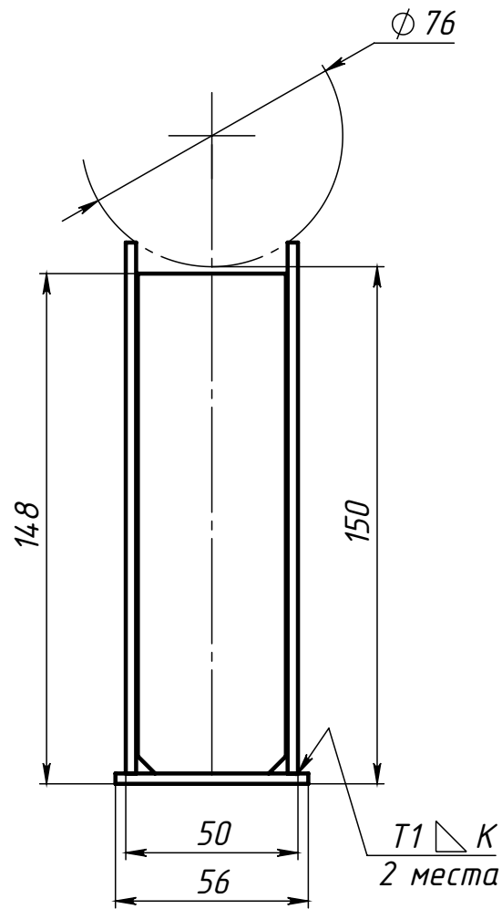
Поз.2 (Ребро)
